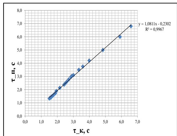
Рисунок 3 – Зависимость постоянных времени, полученных при прямом способе от постоянных времени, полученных при косвенном способе определения постоянной времени термометра
