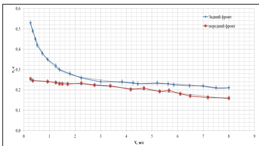
Рисунок 5 – Зависимость \tau = f(V) , полученная при прямом способе воздействия
