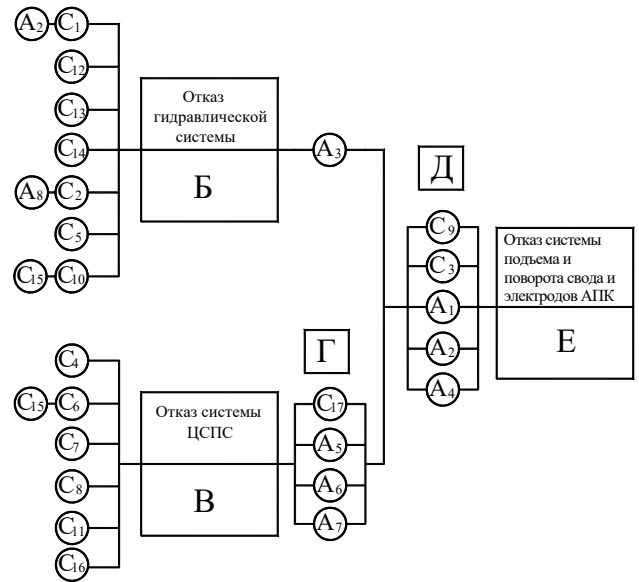
Рисунок 11. Механизм подъема и поворота свода и электродов агрегата печь-ковш (а), дерево отказов механизма подъема и поворота свода и электродов агрегата печь-ковш (б)
