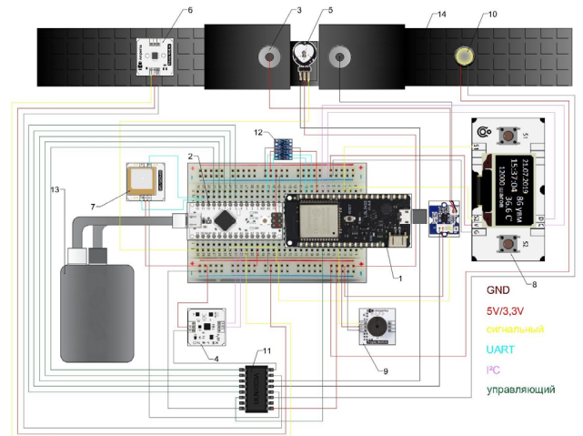
Рисунок 14. Принципиальная схема разработанного носимого устройства
