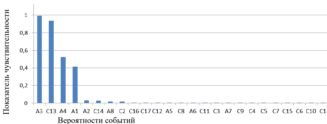
Рисунок 12. Показатели чувствительности отказов технических узлов и ошибок оператора согласно таблице 3
