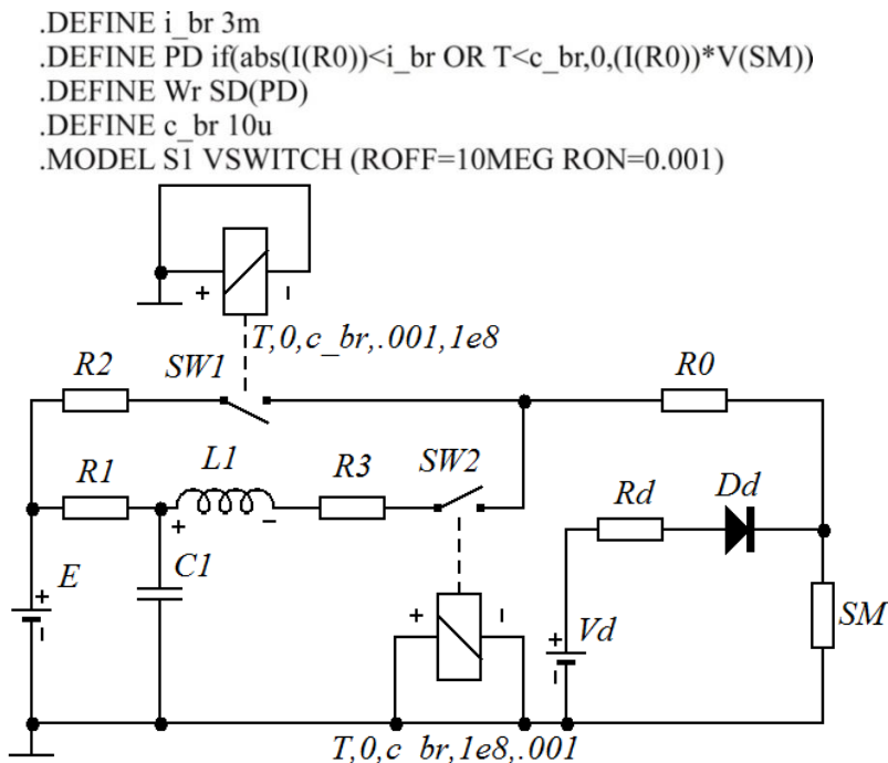
Рисунок 1— Схема компьютерной модели расчёта параметров разряда искробезопасной индуктивно-ёмкостной цепи
