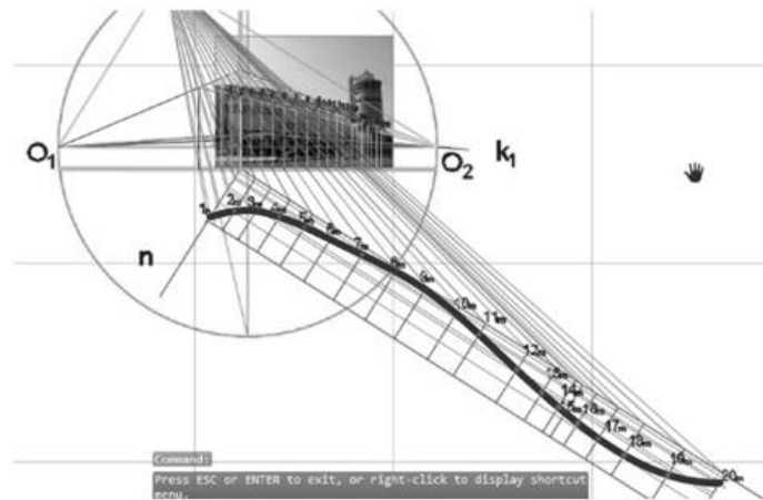
Рисунок 5 – Отыскание относительной натуральной величины кривой линии фасада Донецк-Сити
