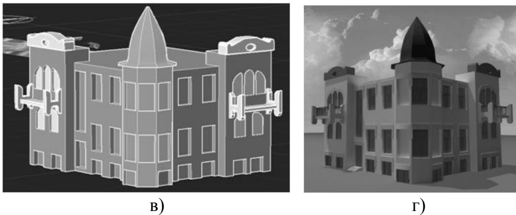
Рисунок 11 – Этапы моделирования дома Горелика: а) отыскание относительных натуральных величин общего блока дома; б) отыскание относительных натуральных величин крыши; в) модель дома в среде AutoCAD; г) визуализация модели дома
