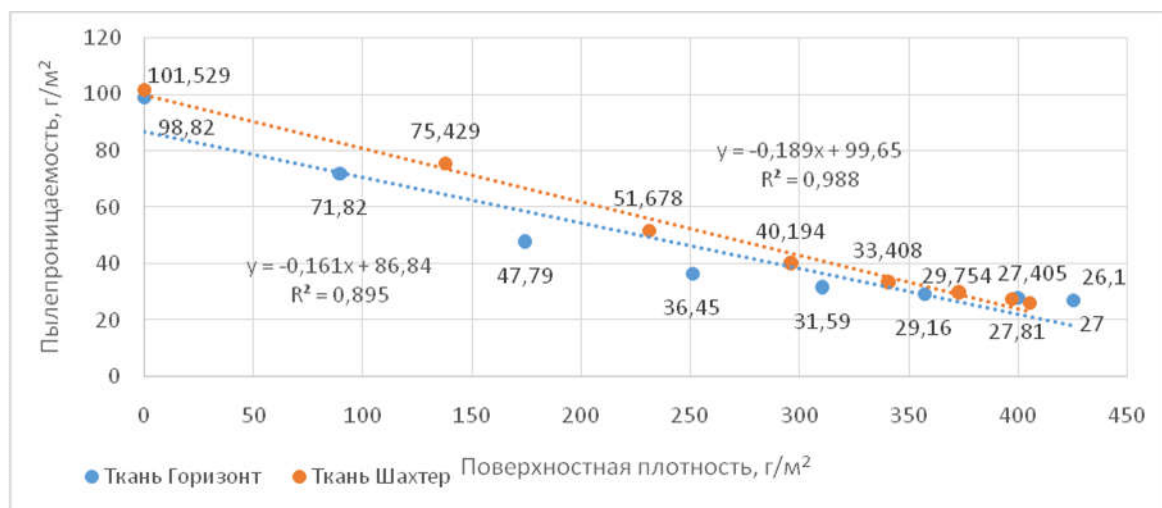
Рисунок 3. Зависимость изменения уровня пылепроницаемости тканей «Горизонт» и «Шахтер» от потери массы.
