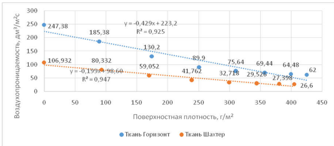
Рисунок 2. Зависимость изменения уровней воздухопроницаемости тканей «Горизонт» и «Шахтер» от потери ее массы.
