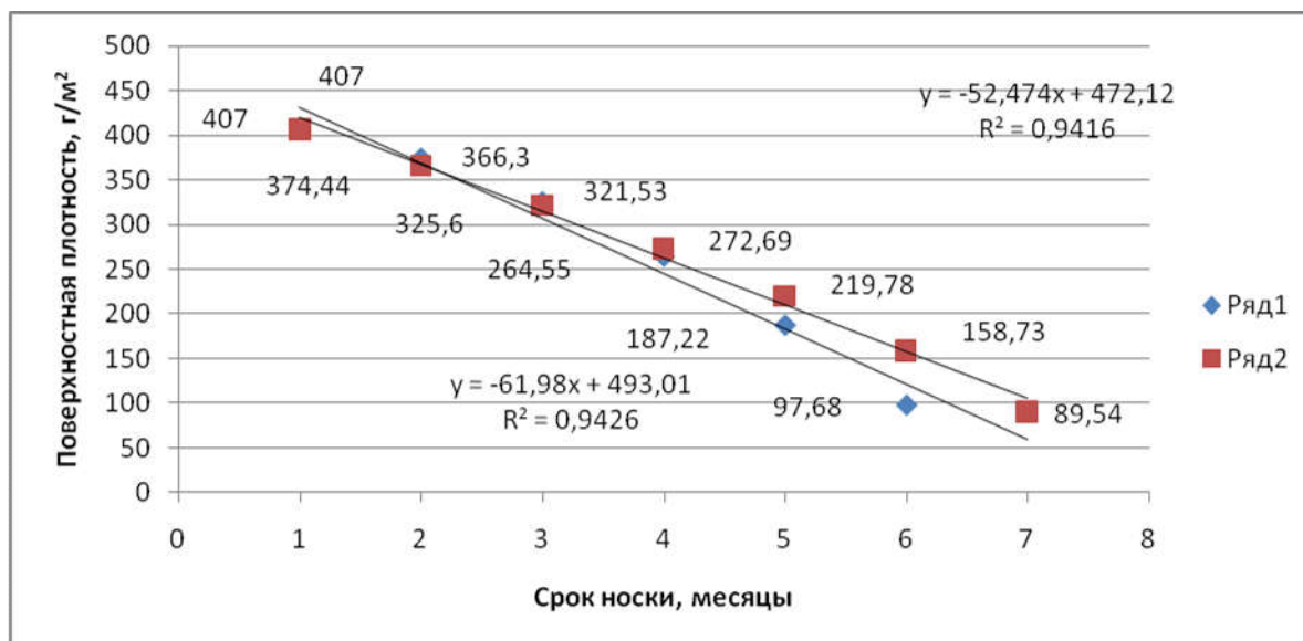
Рисунок 10. Зависимость степени износа спецодежды шахтерской из ткани «Горизонт» при работе на маломощных пластах от срока эксплуатации в области колен (ряд 1), бедра и голени (ряд 2).
