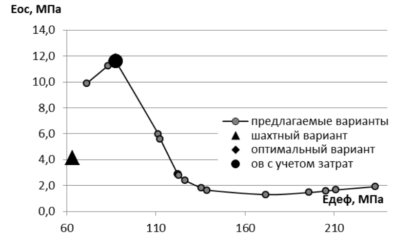
Рисунок 14 - График зависимости эффективности работы охранного сооружения (тумб с распором) по поддержанию выработки E_{ос} , МПа от модуля его деформации E_{деф} , МПа для условий шахты «Щегловская-Глубокая» ( Ш_п = 15м )
