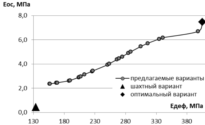
Рисунок 11 - График зависимости эффективности работы охранного сооружения (тумб с распором) по поддержанию выработки E_{ос} , МПа от модуля его деформации E_{деф} , МПа для условий шахты «Рассвет-1» ( Ш_о = 50м )
