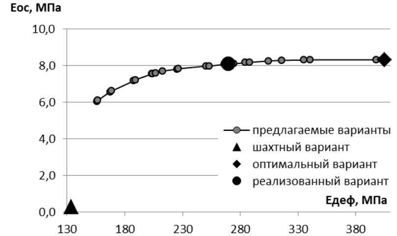
Рисунок 12 - График зависимости эффективности работы охранного сооружения (тумб с распором) по поддержанию выработки E_{ос} , МПа от модуля его деформации E_{деф} , МПа для условий шахты «Рассвет-1» ( Ш_п = 15м )
