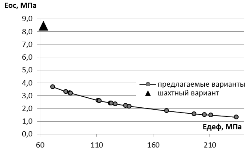
Рисунок 13 - График зависимости эффективности работы охранного сооружения (тумб с распором) по поддержанию выработки E_{ос} , МПа от модуля его деформации E_{деф} , МПа для условий шахты «Щегловская-Глубокая» ( Ш_о = 50м )
