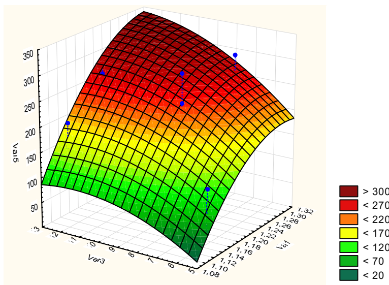
Рисунок 3 – Изменение статической нагрузки ( P_{ст} ) (в природе) от отношений d_a/d_{ш} и E_n/E_a
