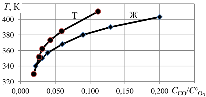
Рисунок 4 – Зависимость температуры самонагрева углей марки Ж и Т от отношения концентраций
