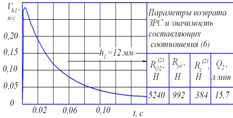
Рисунок 4 – Характер изменения V_{h1} при использовании плунжерного золотника с положительным перекрытием окон штока
